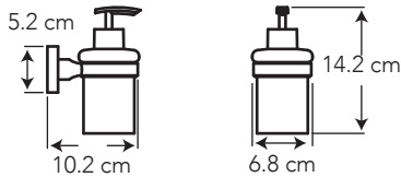
Dispensador de Jabón COD. SG0016630161CW
