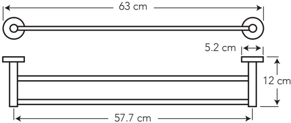
Toallero Doble COD. SG0016670161CW
